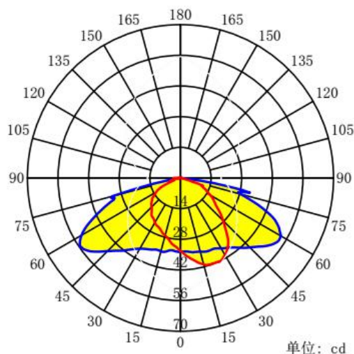
配光曲线
